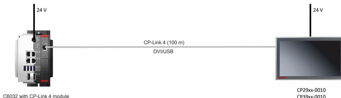
Fig. 12: CP29xx-0010_CP-Link 4
